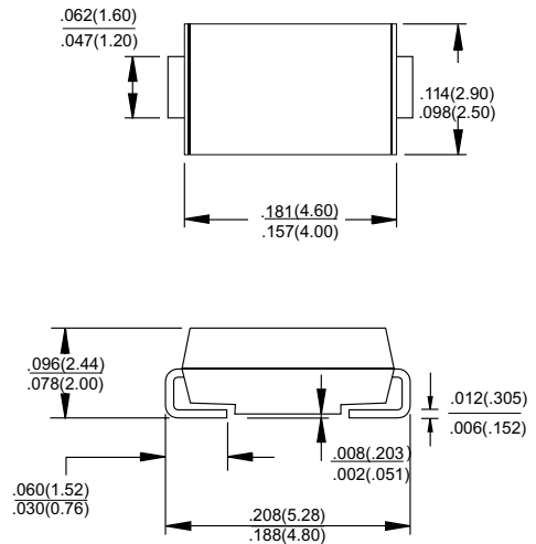
SMA/DO-214AC Unit:inch(mm)
